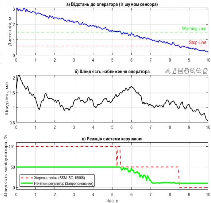
Рис. 3. Результати моделювання реакції системи керування
