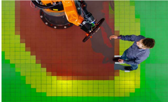
Рис. 1. Принцип дії адаптивної системи безпеки з динамічним масштабуванням зон
