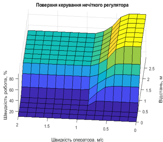
Рис. 4. Поверхня нечіткого виводу синтезованого регулятора
