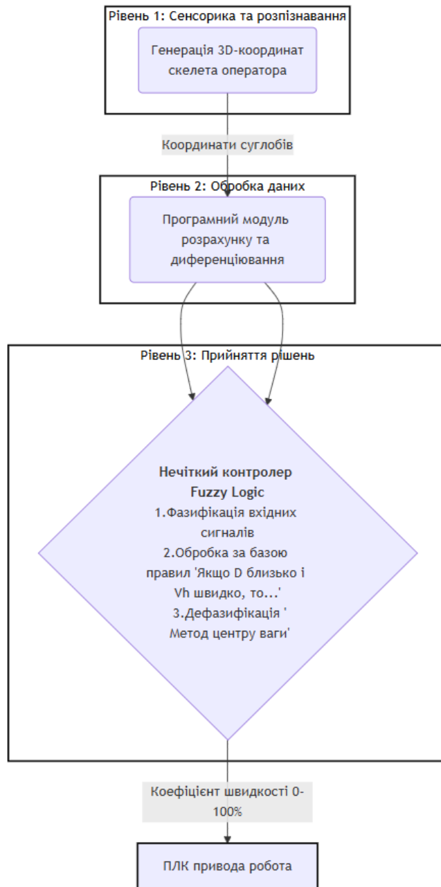
Рис. 2. Блок-схема архітектури розглянутої інтелектуальної системи безпеки
